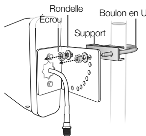
Ensemble d'antenne extérieure
